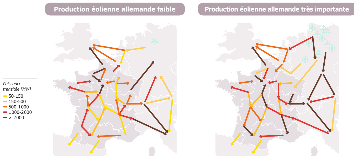
Figure 1.5 Influence de la production éolienne en Allemagne sur les flux sur le réseau en France
