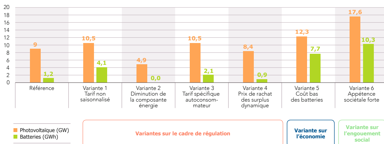
Figure 1.6 Estimations du développement de l'autoconsommation individuelle dans le secteur résidentiel dans le scénario Ampère à l'horizon 2035 selon différentes variantes ( analyses du Bilan prévisionnel 2017 )
