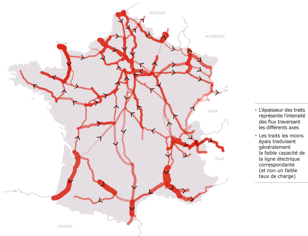
Figure 1.3 Illustration des flux sur le réseau de grand transport et les réseaux régionaux
