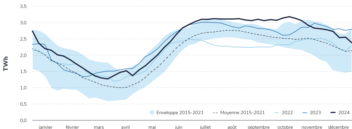
Figure 2.9 : Évolution hebdomadaire du stock hydraulique au cours de l'année 2024 en France et comparaison avec les années précédentes
