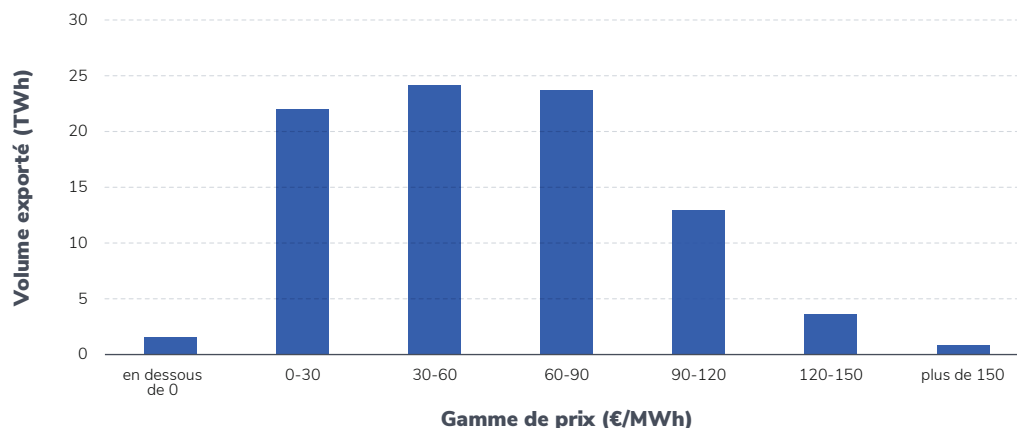
Figure 4.20 - Distribution des exportations de la France en fonction de la gamme de prix spot français en 2024
