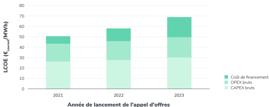
Figure 2.16 : Évolution des coûts complets de production éoliens terrestres
