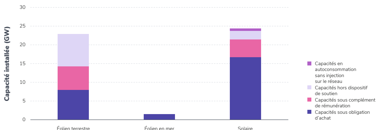
Figure 2.26 : Répartition des capacités éoliennes et solaires selon la modalité de valorisation de leur production
