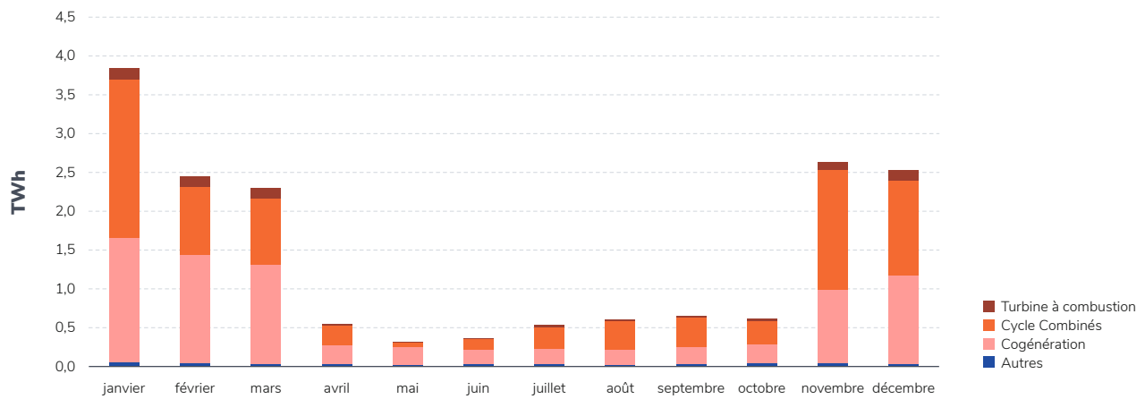
Figure 2.31 : Évolution de la production mensuelle des centrales à gaz en France et décomposition par type de centrale en 2024
