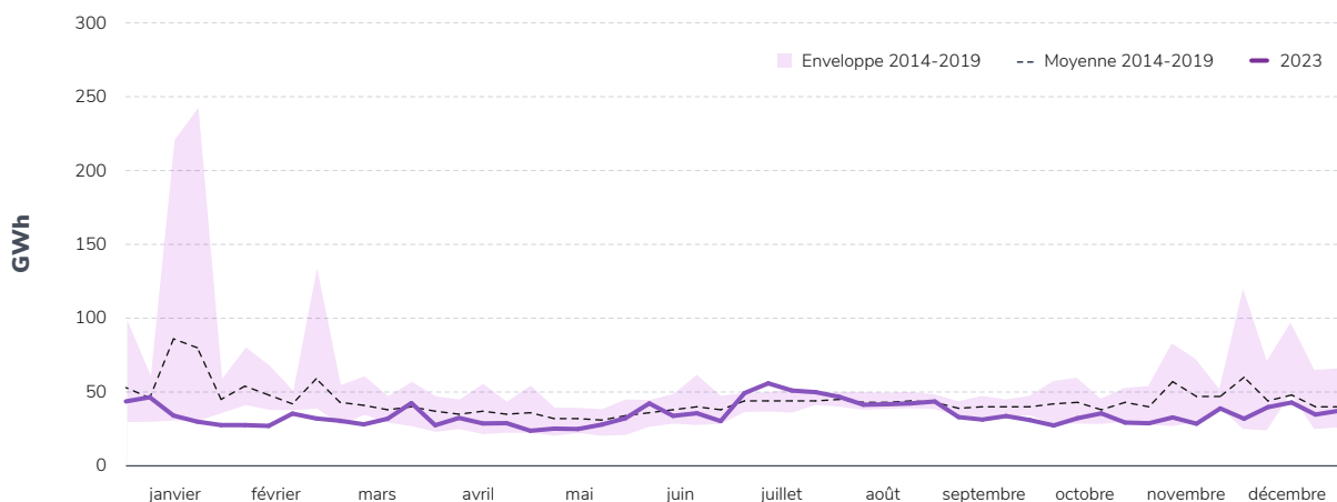
Figure 2.33 : Évolution de la production hebdomadaire des centrales au fioul en France au cours de l'année 2024 et comparaison avec les années précédentes
