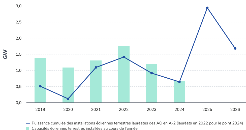
Figure 2.17 : Mise en perspective de l'évolution du parc éolien terrestre avec la puissance cumulée des lauréats des appels d'offres de la CRE
