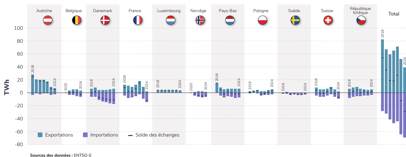
Figure 6.11 : Échanges commerciaux entre l'Allemagne et les pays voisins
