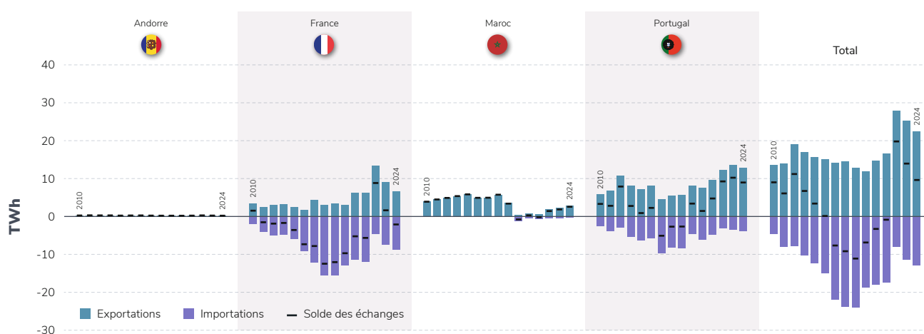
Figure 6.35 : Échanges commerciaux d'électricité entre l'Espagne et ses voisins
