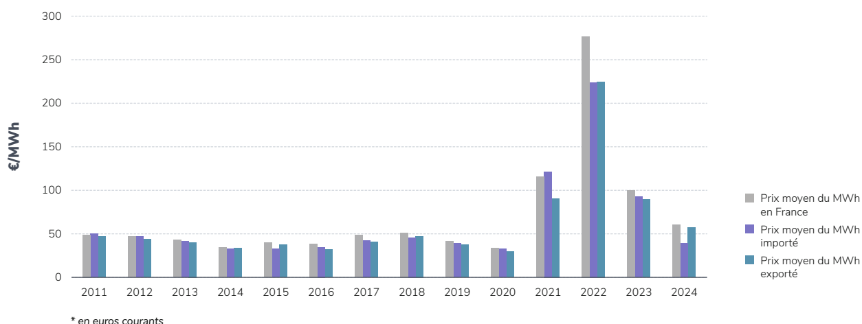
Figure 4.21 - Prix moyen du MWh exporté, importé et produit en France, entre 2011 et 2024
