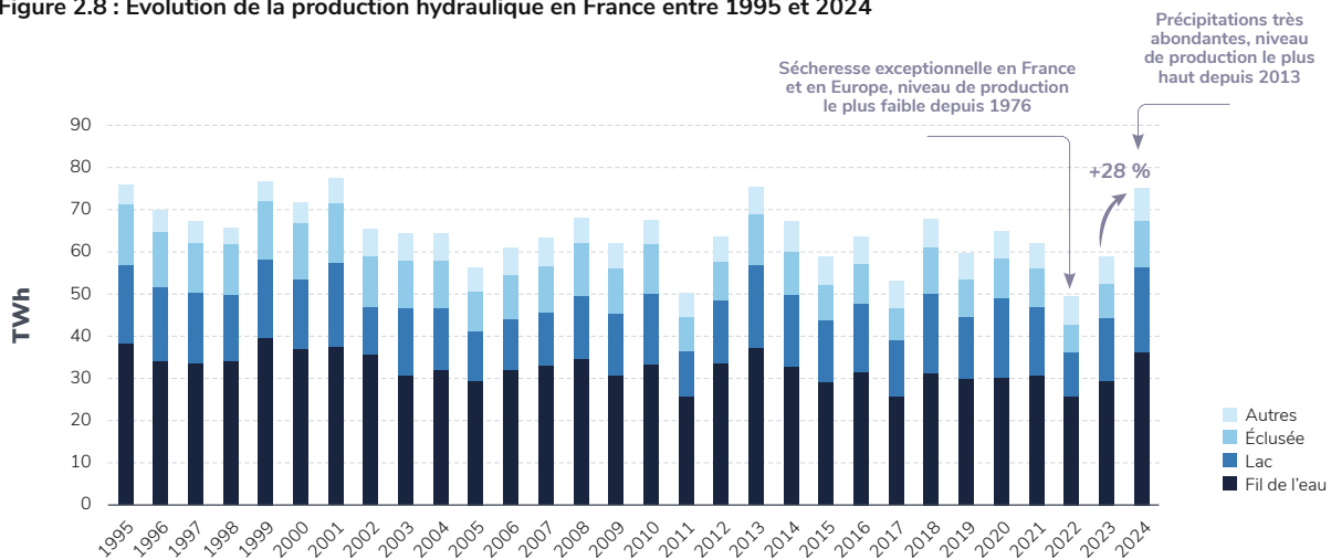
Figure 2.8 : Évolution de la production hydraulique en France entre 1995 et 2024
