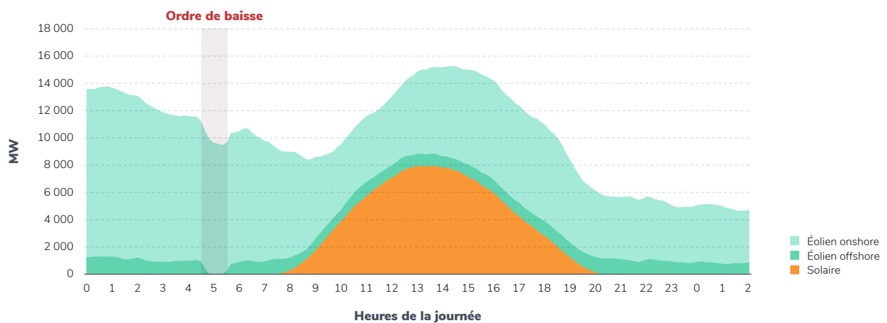
Figure 2.27 : Production éolienne et solaire au cours de la journée du 11 septembre 2024
