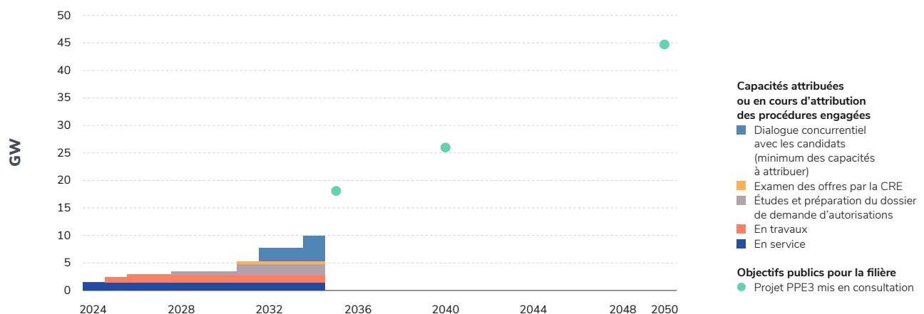
Figure 2.19 : Mises en service des capacités éoliennes en mer prévues à fin 2024
