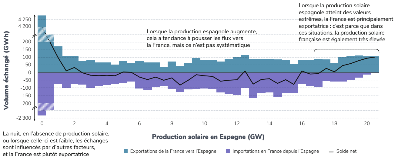
Figure 4.9 - Volume échangé entre la France et l'Espagne en 2024 en fonction de la production solaire espagnole
