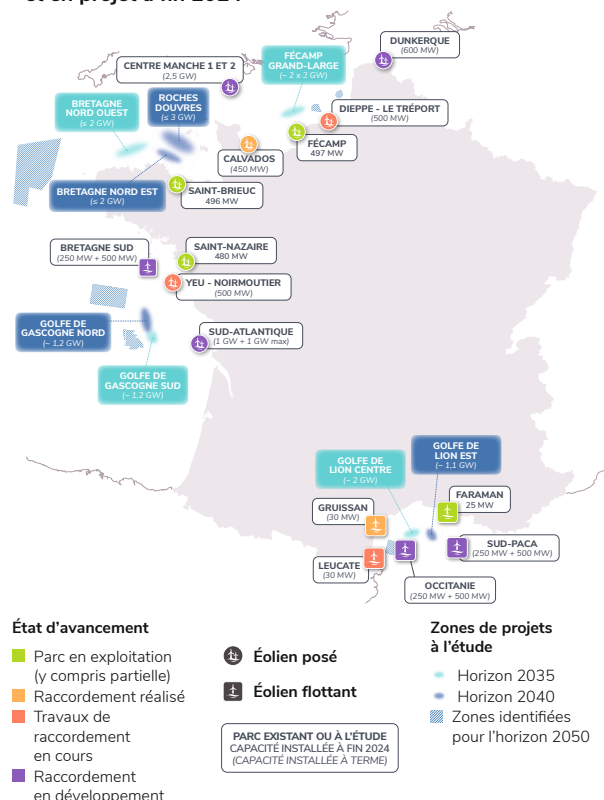
Figure 2.18 : Carte des parcs éoliens en mer existants et en projet à fin 2024
