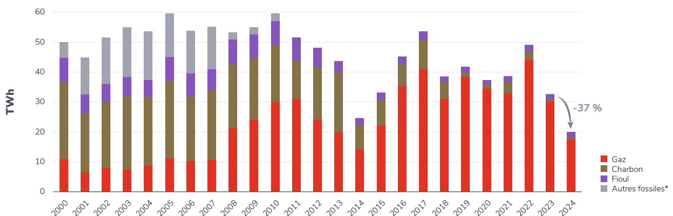
Figure 2.29 : Évolution de la production thermique fossile en France depuis 2001
