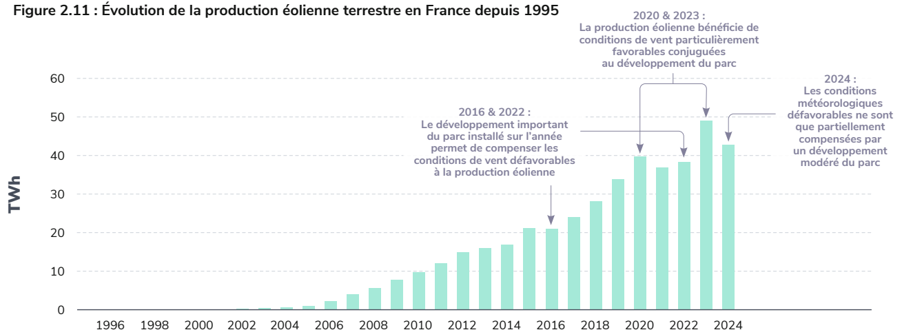
Figure 2.11 : Évolution de la production éolienne terrestre en France depuis 1995
