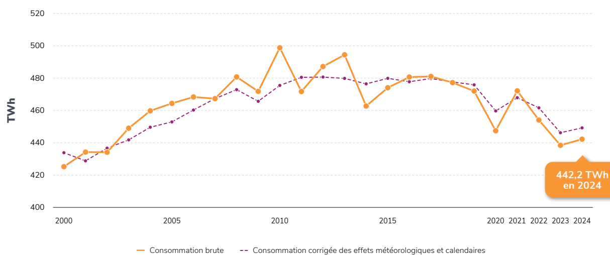
Figure 1.8 - Évolution de la consommation non corrigée des aléas météorologiques depuis 2000.
