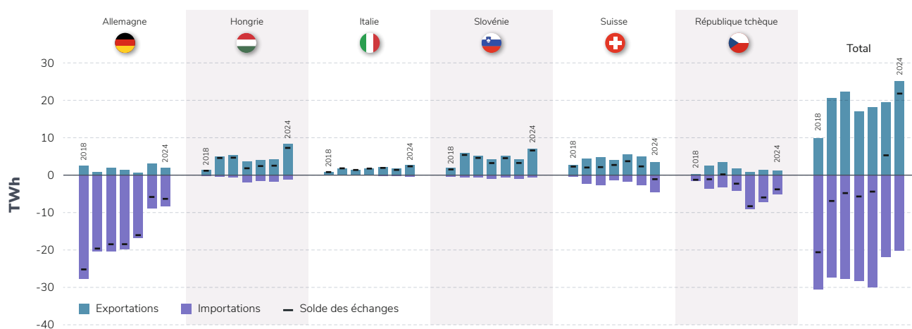
Figure 6.31 : Échanges commerciaux d'électricité entre l'Autriche et ses voisins
