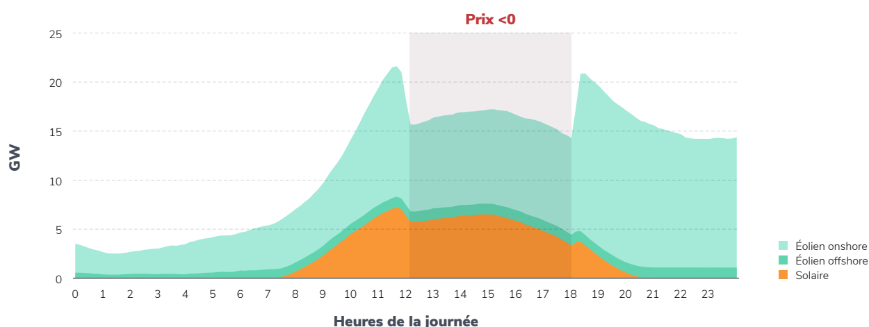
Figure 25 : Production éolienne et solaire du 15 avril 2024 (prix spot négatif de 12 h à 17 h)
