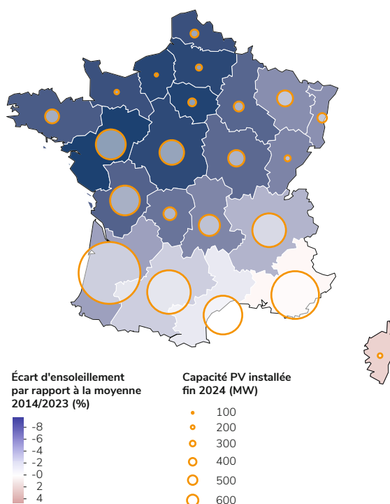
Figure 2.22 : Déficit d'ensoleillement en France au cours de l'année 2024 par rapport à la moyenne 2014-2023
