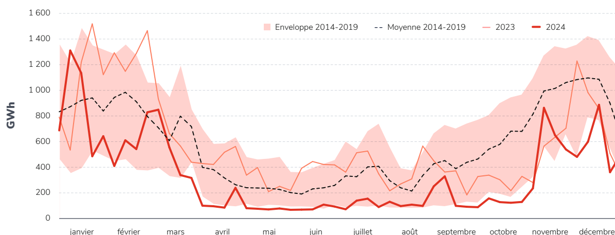
Figure 2.30 : Évolution de la production hebdomadaire des centrales à gaz en France au cours de l'année 2024 et comparaison avec les années précédentes
