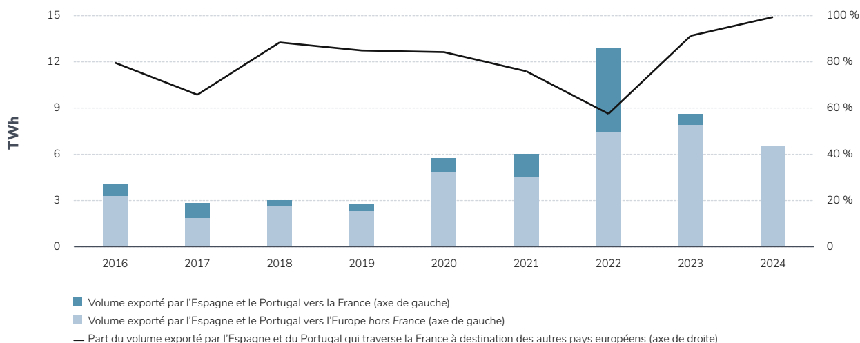
Figure 4.18 - Exportations depuis la péninsule ibérique vers la France et le reste de l'Europe
