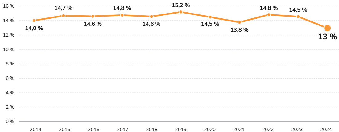
Figure 2.21 : Facteur de charge annuel du parc photovoltaïque en France entre 2014 et 2024
