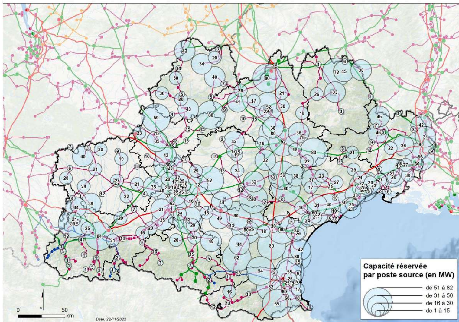
Carte des Capacités réservées par poste
