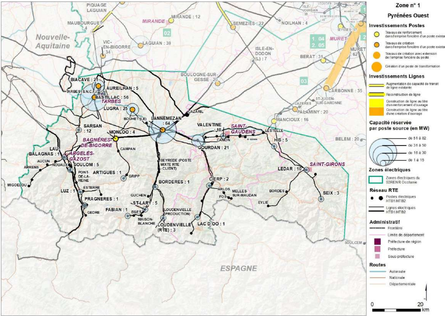
La carte ci-après récapitule les capacités réservées sur chacun des postes électriques et les projets envisagés sur le réseau électrique dans la zone 1 [Pyrénées Ouest]
