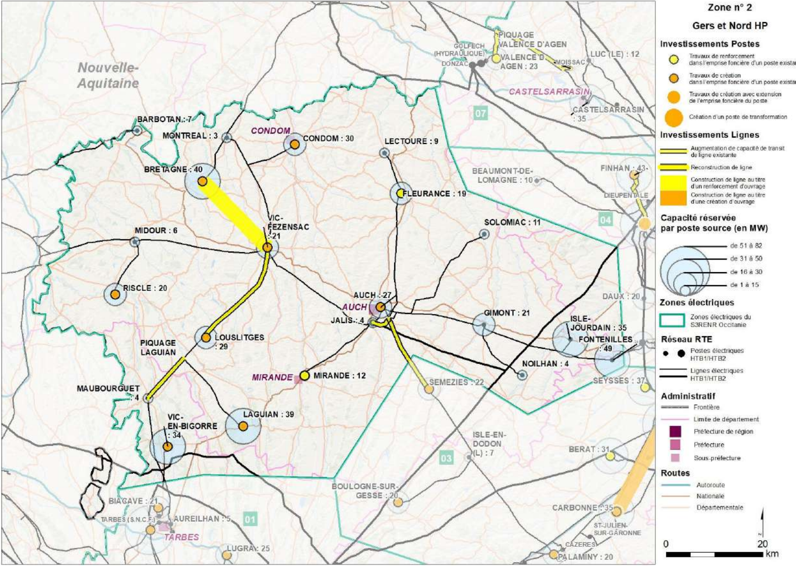
La carte ci-après récapitule les capacités réservées sur chacun des postes électriques et les projets envisagés sur le réseau électrique dans la zone 2 [Gers et Nord Hautes-Pyrénées]
