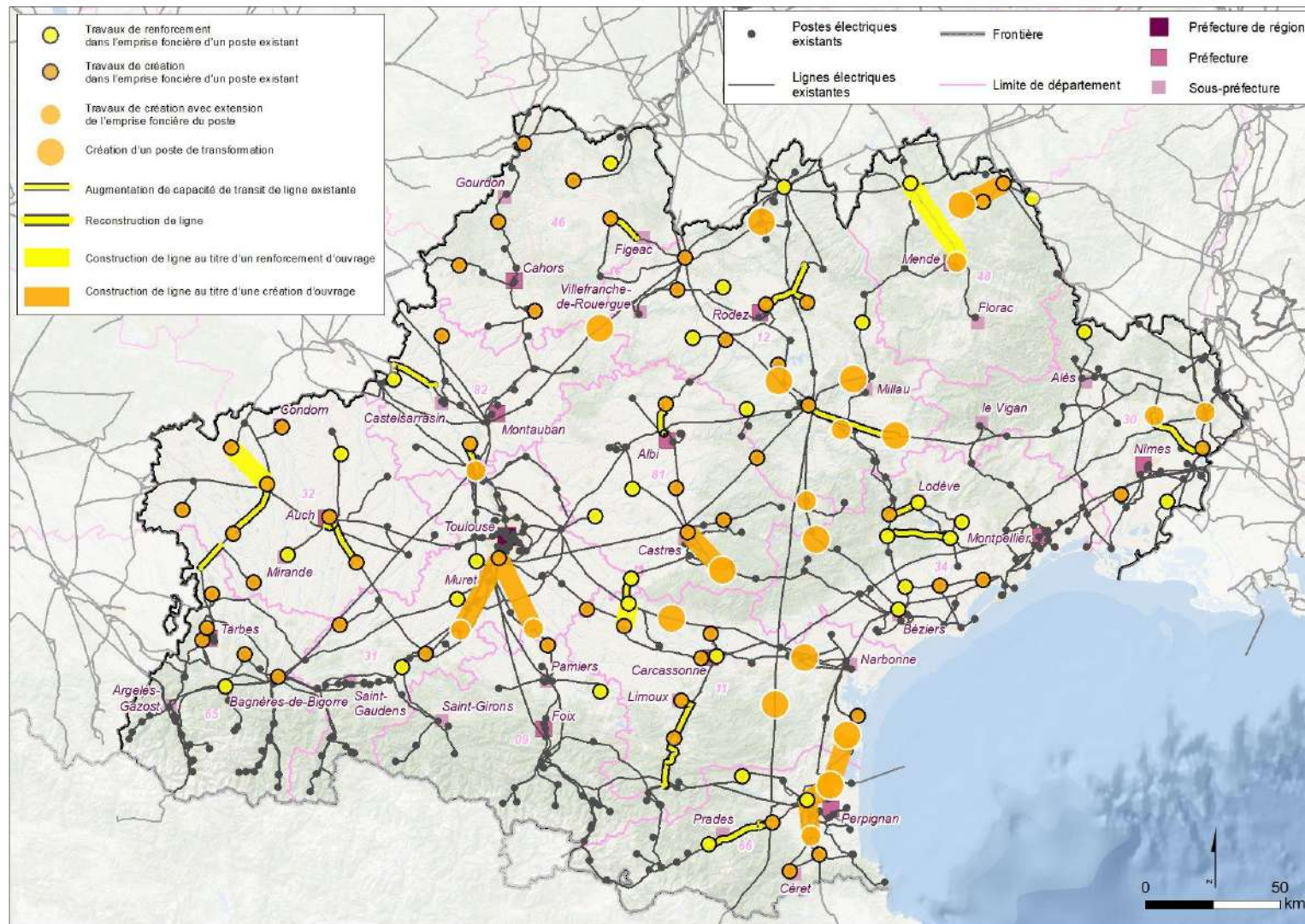
Carte des investissements prévus par le S3REnR Occitanie
