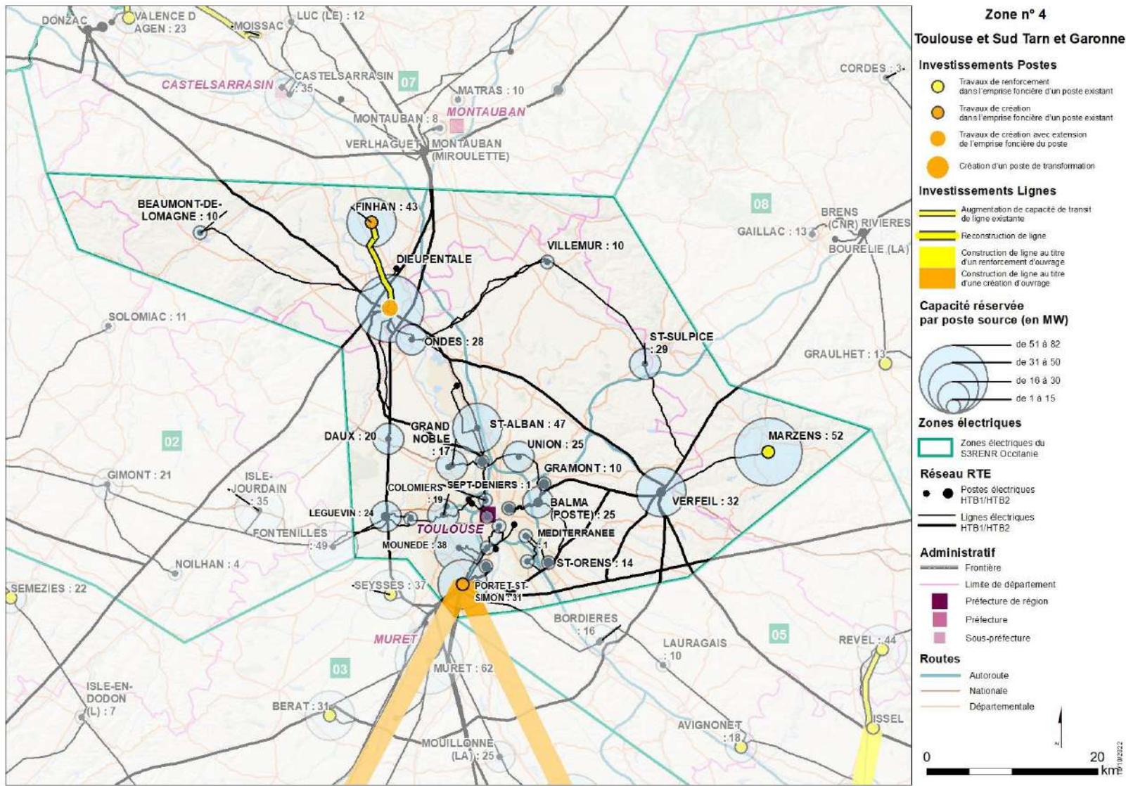
La carte ci-après récapitule les capacités réservées sur chacun des postes électriques et les projets envisagés sur le réseau électrique dans la zone 4 [Toulouse et Sud Tarn-et-Garonne]
