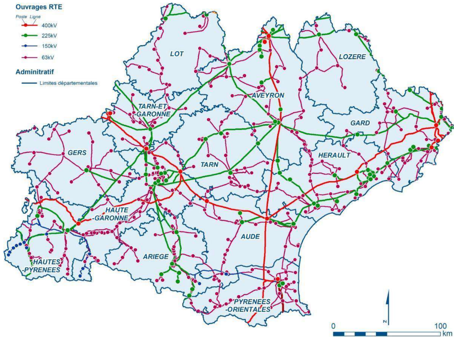
Le réseau public de transport d'électricité existant en région Occitanie
