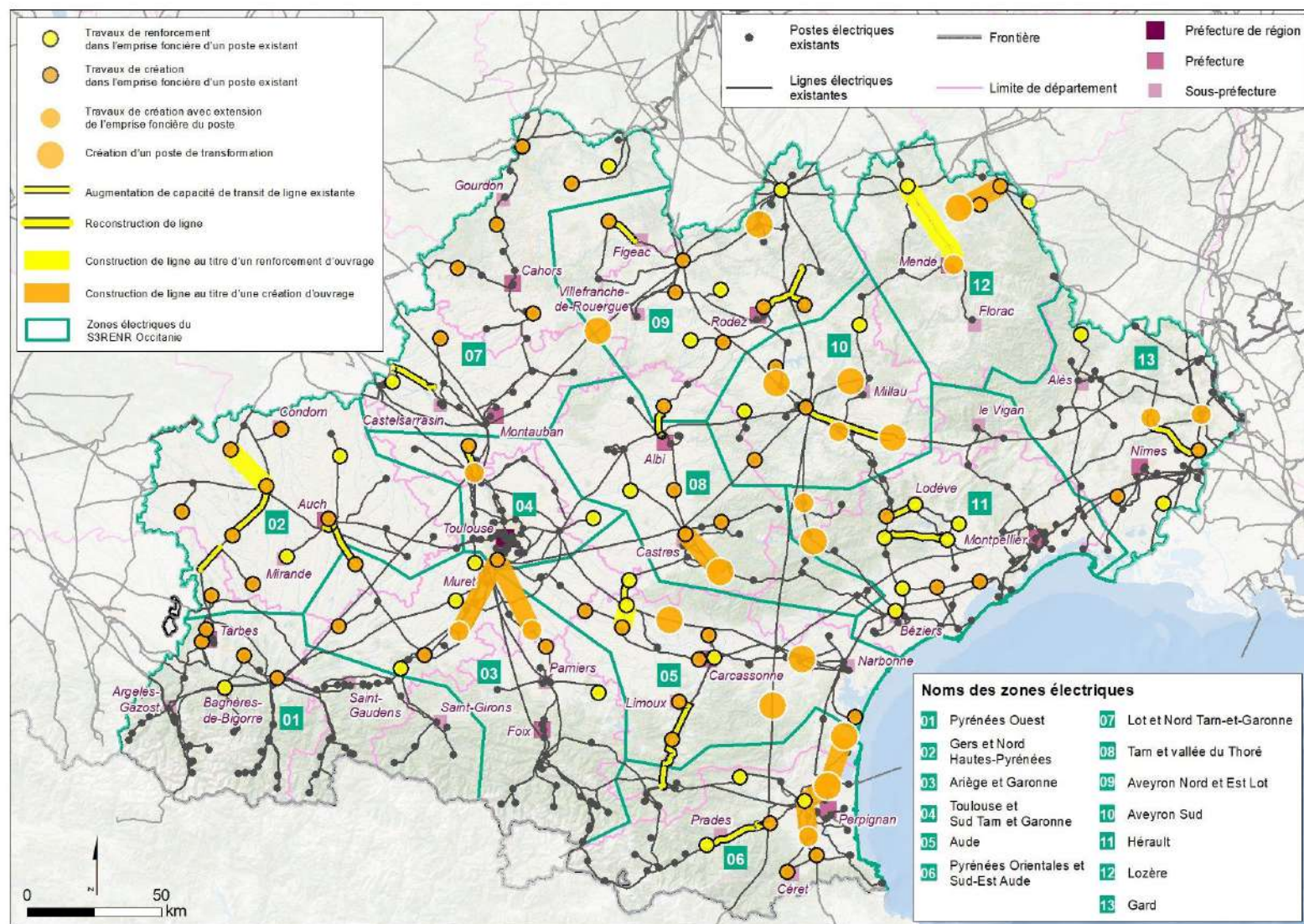
Figure 8 : Carte des investissements prévus dans le S3REnR Occitanie et découpage en zones électriques
