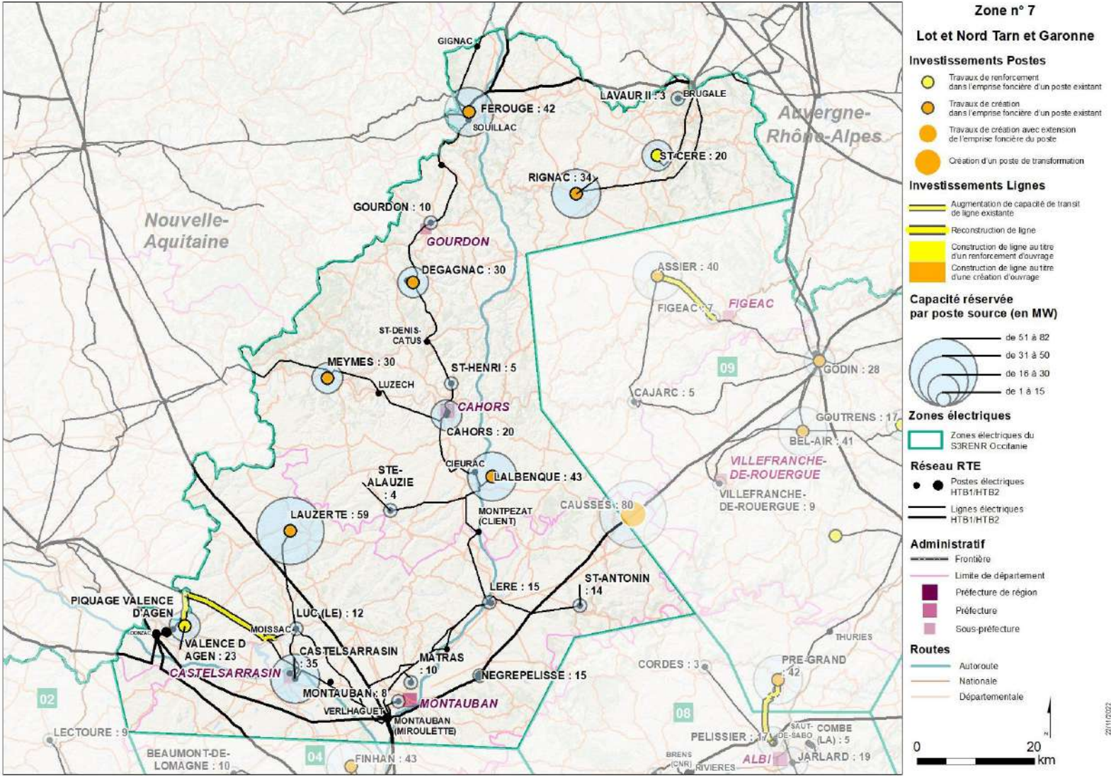
La carte ci-après récapitule les capacités réservées sur chacun des postes électriques et les projets envisagés sur le réseau électrique dans la zone 7 [Lot et Nord Tarn et Garonne]
