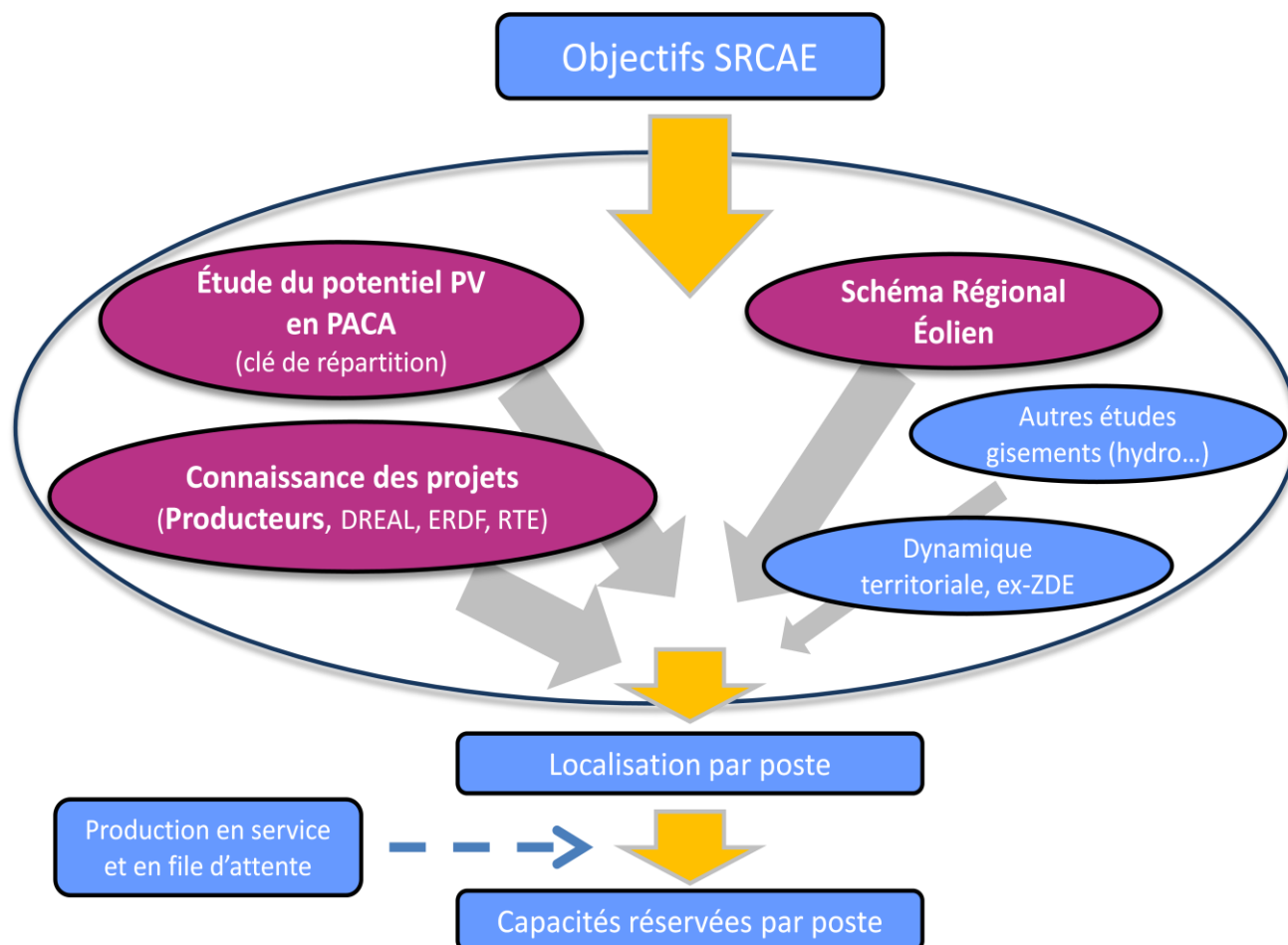
Schématisme de la méthodologie de réservation de capacités sur le réseau électrique
