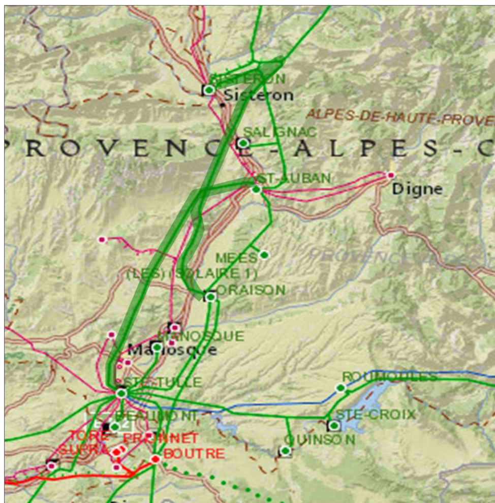
Les aménagements de réseau proposés dans le S3REnR en moyenne Durance
