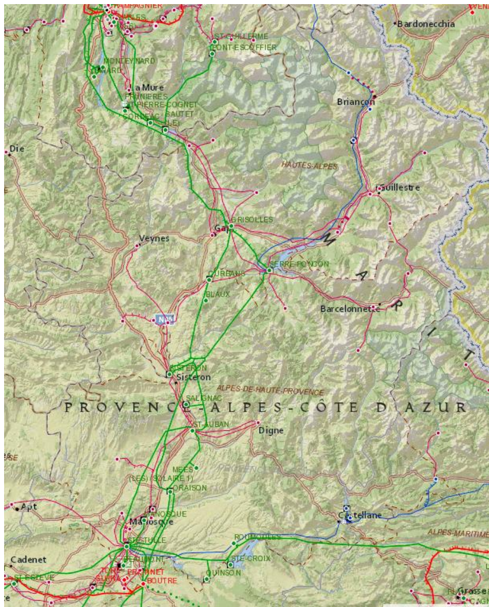
Le réseau électrique Très Haute Tension en Durance
