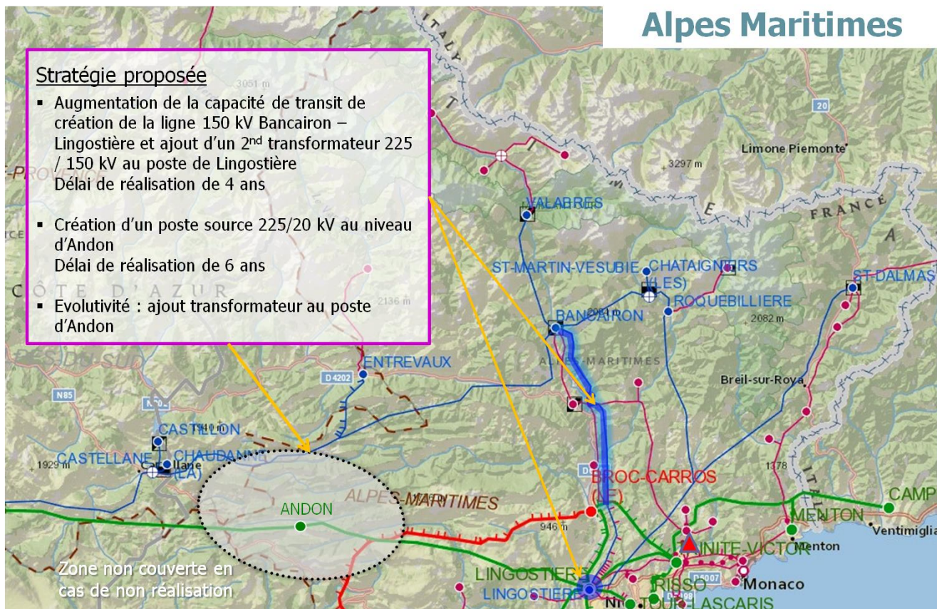
Evolutions du réseau dans les Alpes Maritimes proposées dans le S3REnR
