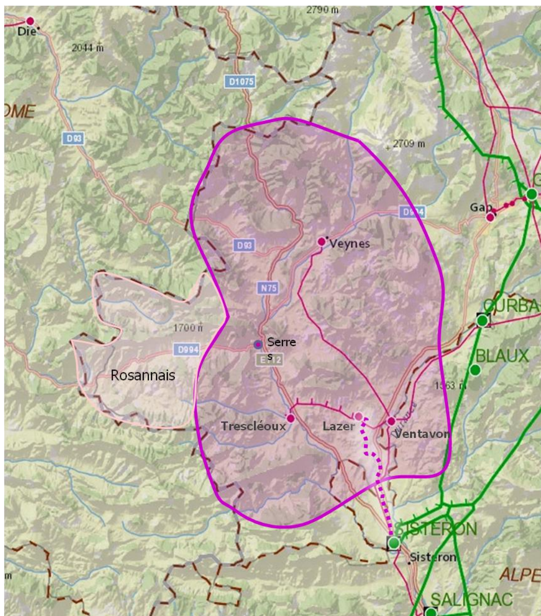
Evolution du réseau 63 kV dans le Buëch dans le cadre du S3REnR.
