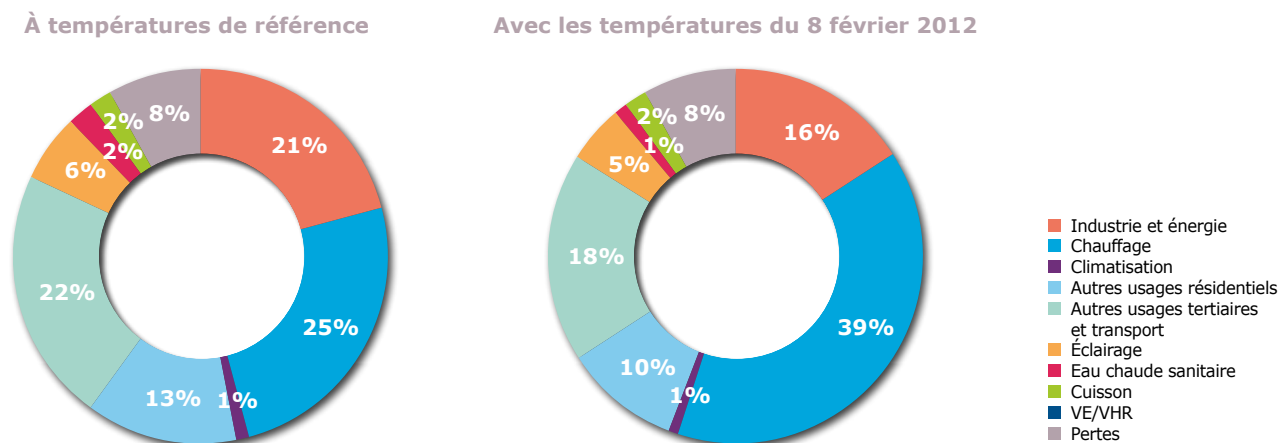
Figure 2.7 Répartition par usages de la puissance appelée entre 8h et 22h un jour ouvré d'hiver
