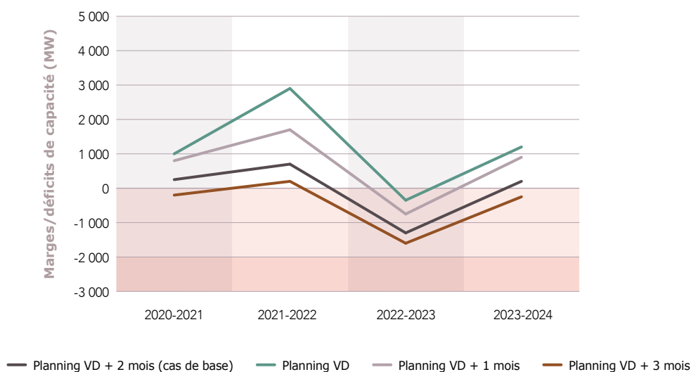
Figure 7.3 Évolution des marges dans le cas de base et selon la tenue du planning des visites décennales
