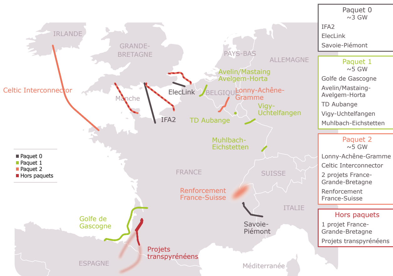
Figure 4.4 Illustration des trois paquets d'interconnexions aux frontières françaises définis dans le SDDR 2019
