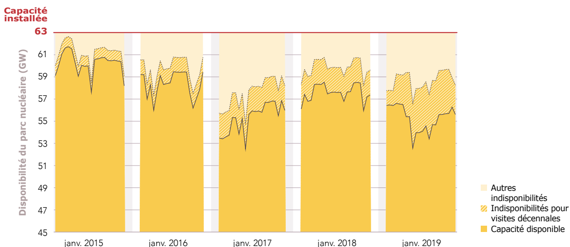
Figure 3.11 Disponibilité du parc nucléaire lors des jours ouvrés en janvier (2015-2019)
