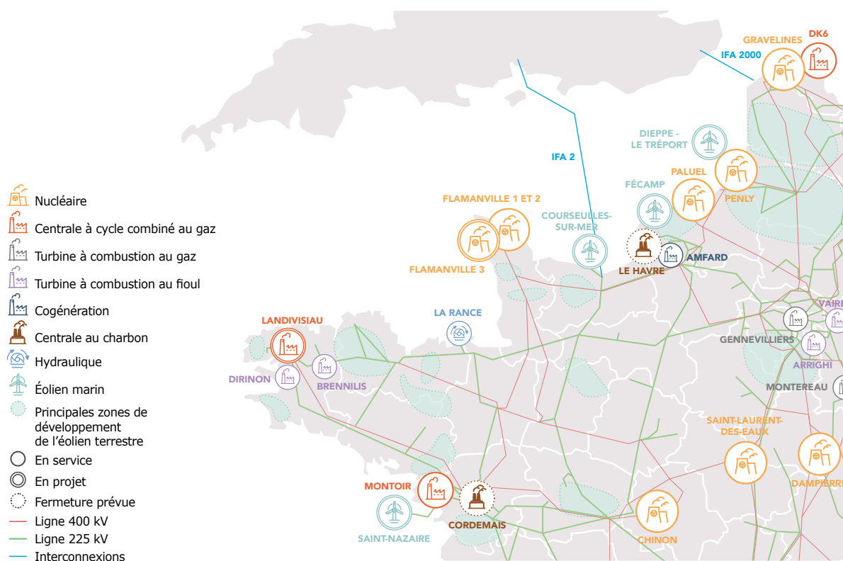
Figure 1.3 Carte du réseau de transport et des principaux moyens de production sur la zone du Grand Ouest
