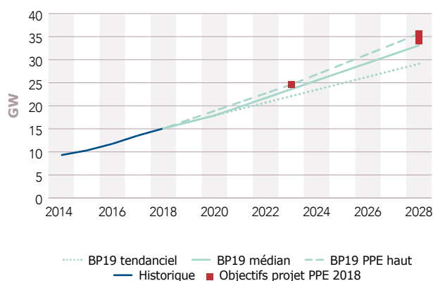
Figure 3.2 Historique et hypothèses d'évolution de la capacité installée de la filière éolienne terrestre au 31 décembre
