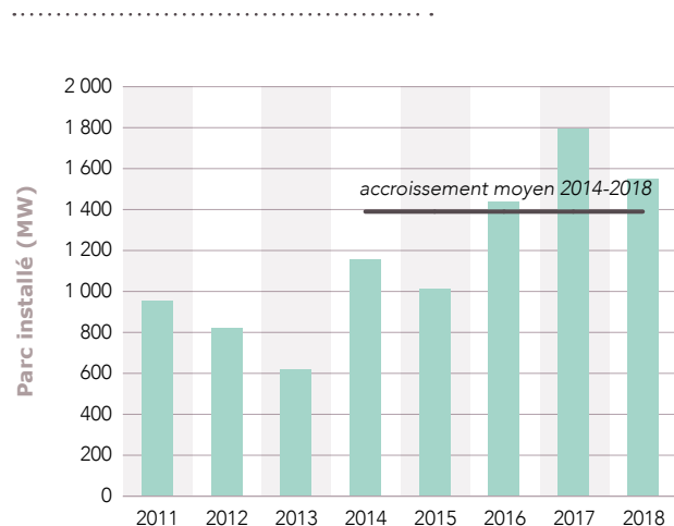
Figure 3.1 Parc installé par année pour la filière éolienne terrestre
