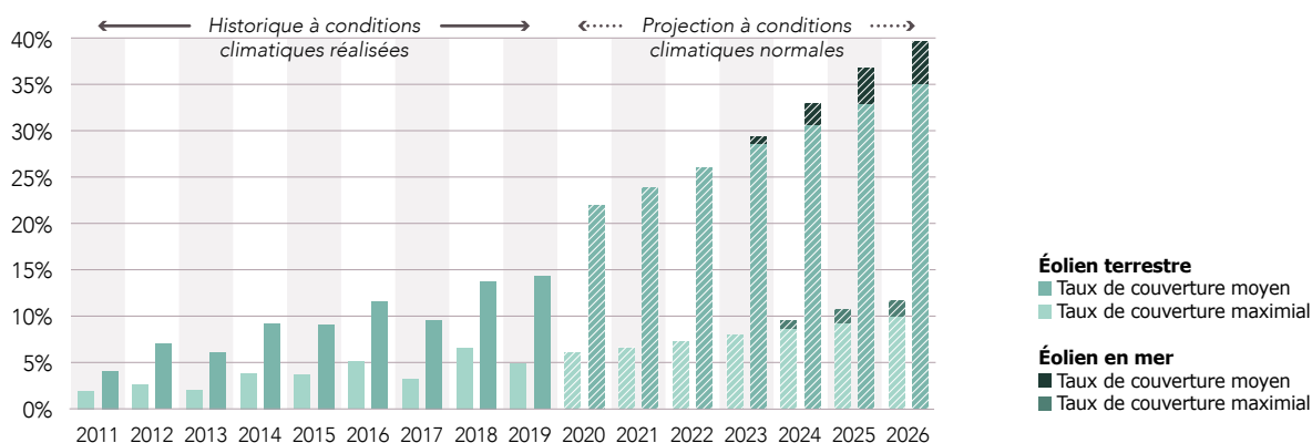
Figure 8.13 Taux de couverture de la pointe de consommation journalière par l'éolien en janvier à 19h
