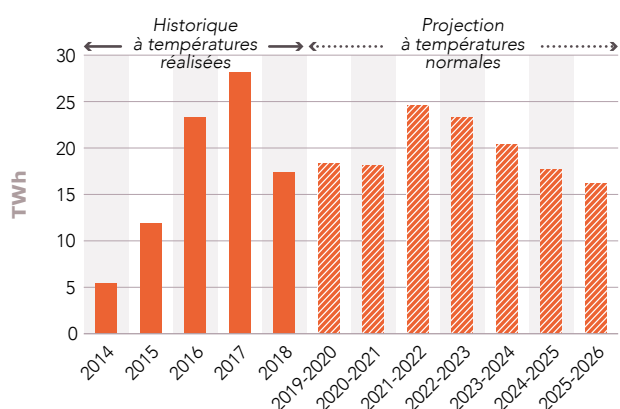
Figure 8.6 Évolution de la production des centrales à cycle combiné au gaz en France
