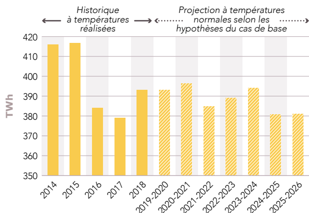
Figure 8.3 Évolution projetée de la production du parc nucléaire en France 63
