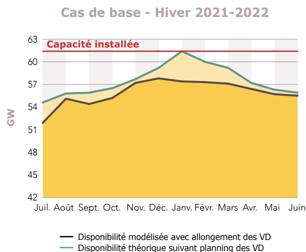
Figure 3.10 Disponibilité théorique moyenne mensuelle considérant uniquement les arrêts pour visite décennale
