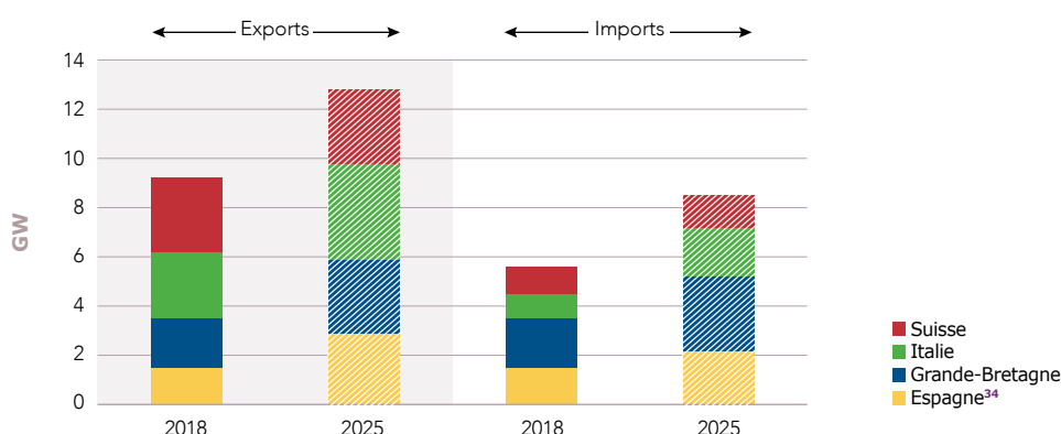
Figure 4.3 Capacités d'échange aux frontières françaises en 2018 et hypothèses en 2025, hors CWE 33
