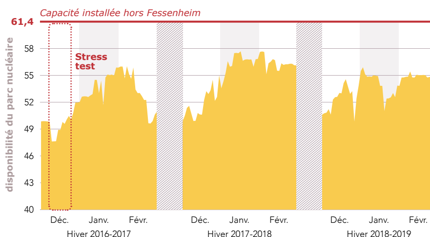
Figure 5.16 Disponibilité moyenne journalière lors des jours ouvrés, hors Fessenheim
