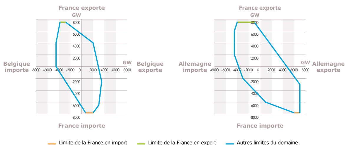
Figure 4.5 Représentation du domaine Flow-Based d'une des journées types hivernales à 19h
