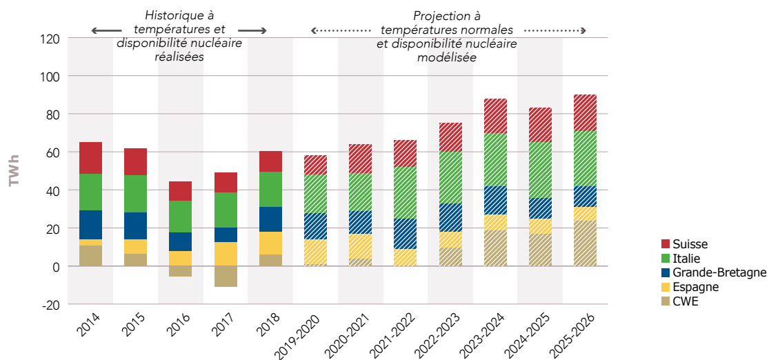
Figure 8.9 Solde des échanges aux frontières françaises en 2018 et en 2025
