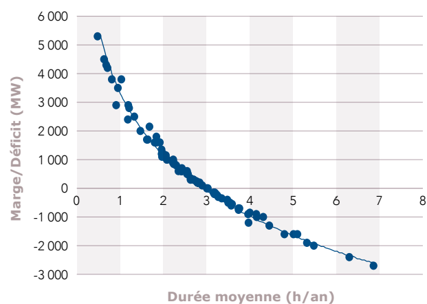
Figure 5.6 Relation entre durée de défaillance et marge ou déficit de capacité
