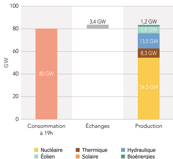
Figure 8.14 Mix de production et échanges moyens à 19h en janvier (en jours ouvrés) Cas de base – 2021
