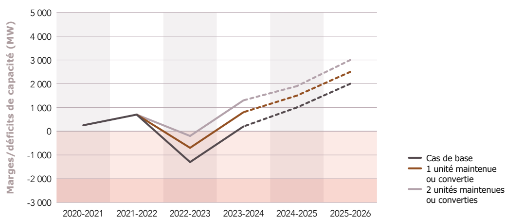
Figure 7.5 Évolution des marges dans un scénario avec maintien ou conversion à la biomasse des deux unités de Cordemais à la biomasse
