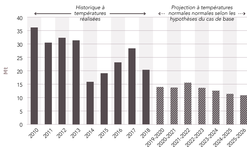
Figure 8.10 Évolution des émissions de CO 2 liées à la production d'électricité en France métropolitaine
