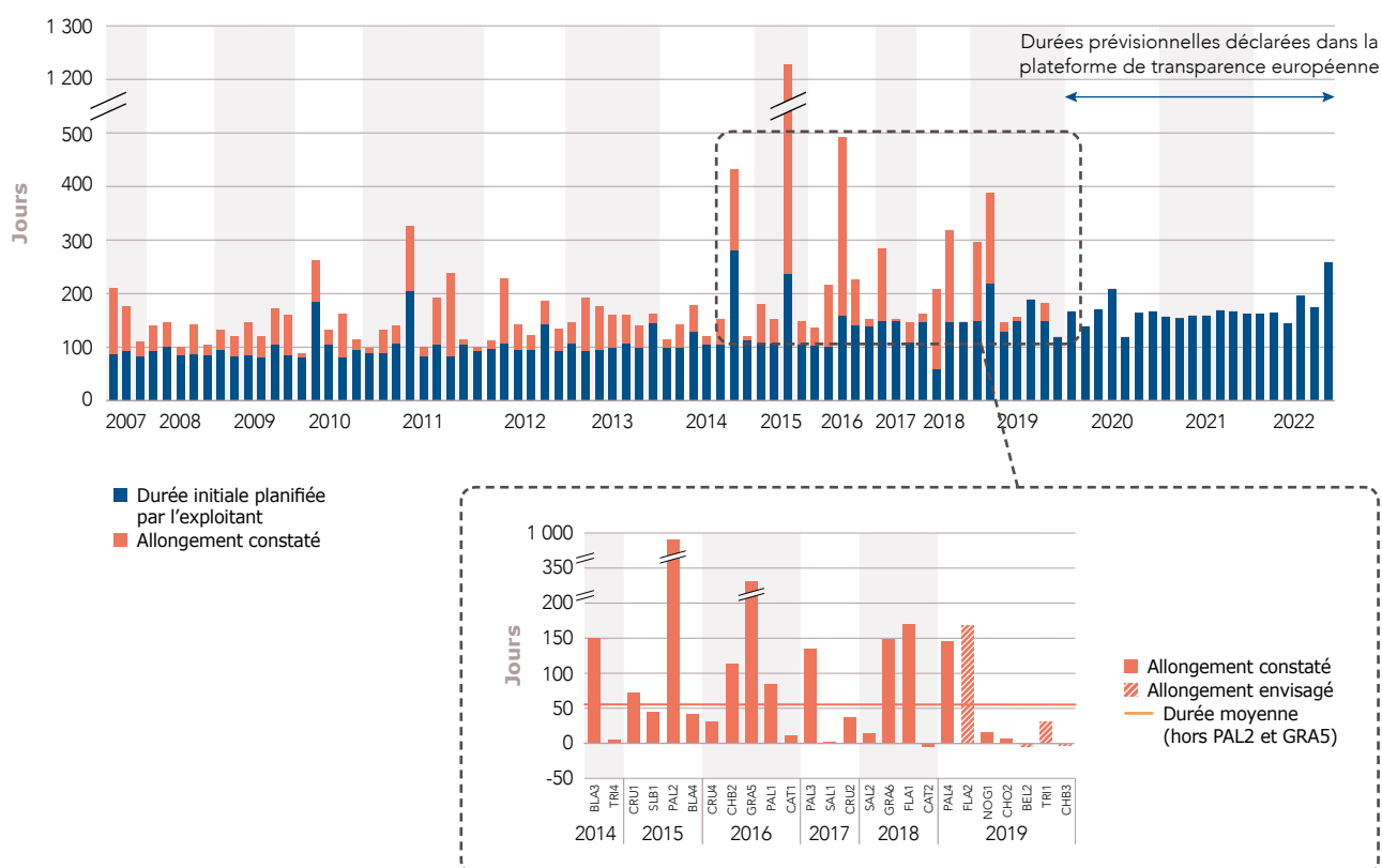
Figure 3.9 Durées initiales planifiées par l'exploitant et allongements constatés au 1 er novembre 2019
