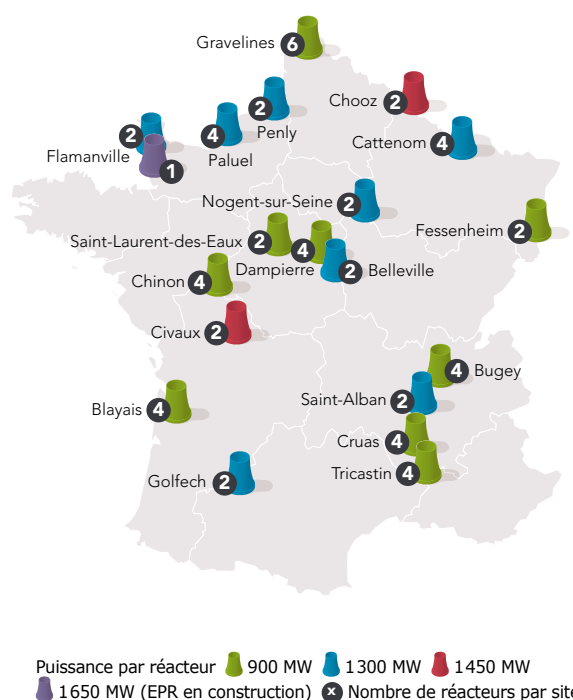
Figure 3.8 Parc nucléaire au 31 décembre 2018
