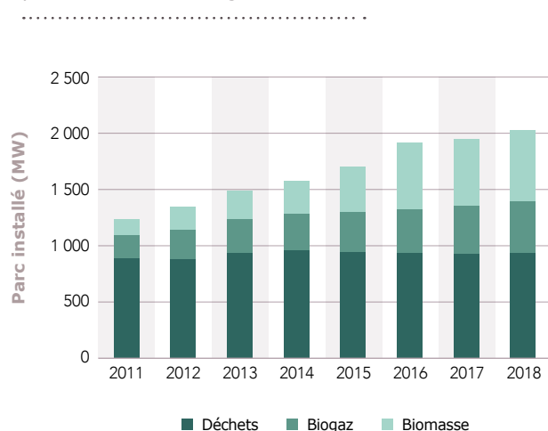
Figure 3.6 Évolution de la capacité installée pour la filière bioénergies
