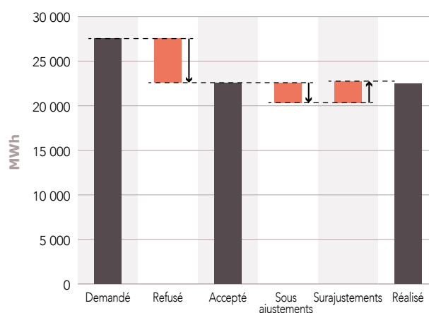
Figure 3.19 Volumes d'effacements demandés et réalisés sur le mécanisme d'ajustement en 2018
