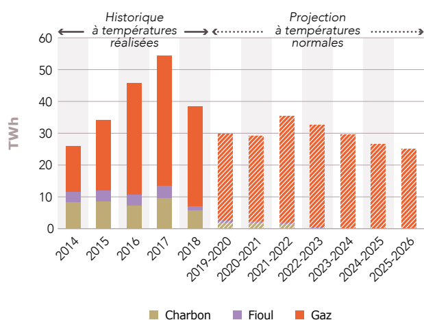
Figure 8.5 Évolution de la production thermique fossile en France
