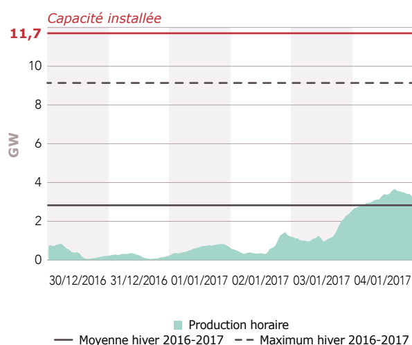
Figure 5.18 Production éolienne horaire en France du 30 décembre 2016 au 4 janvier 2017
