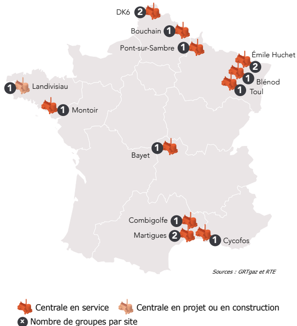
Figure 3.16 Centrales à cycle combiné au gaz au 31 décembre 2018
