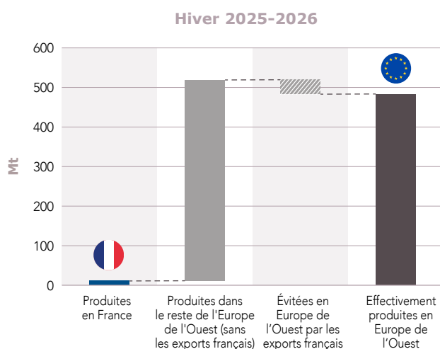
Figure 8.12 Effets du système électrique français sur les émissions annuelles de CO 2 du mix électrique dans les pays européens modélisés dans le Bilan prévisionnel
