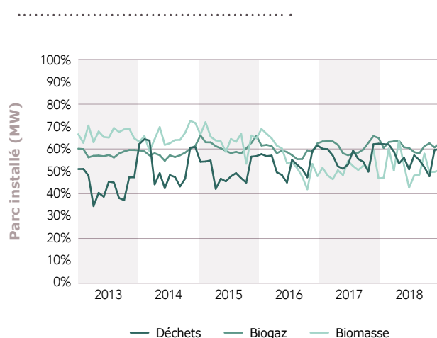
Figure 3.7 Facteurs de charge de la filière bioénergies de 2013 à 2018
