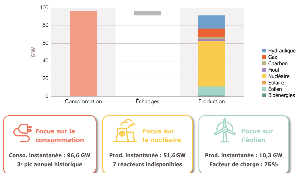
Figure 8.16 Mix de production observé le 28 février 2018 à 19h
