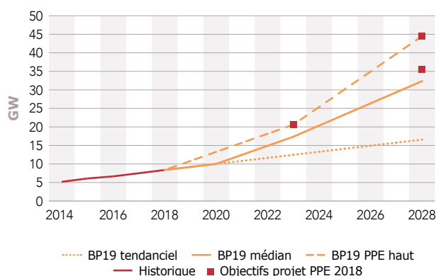
Figure 3.5 Historique et hypothèses d'évolution de la capacité installée pour la filière photovoltaïque au 31 décembre
