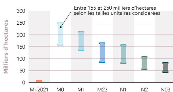
Projection du nombre d'hectares occupés par des panneaux photovoltaïques au sol à l'horizon 2050
