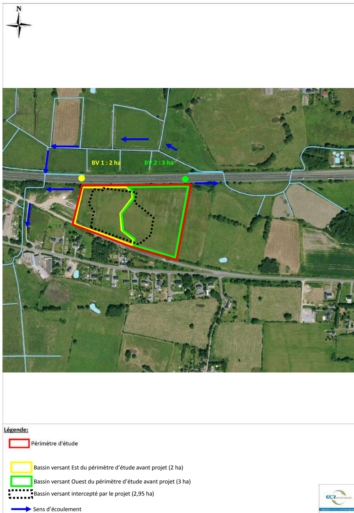
Figure 143 : bassin versant du site d'étude et bassin versant intercepté par le projet (ECR)
