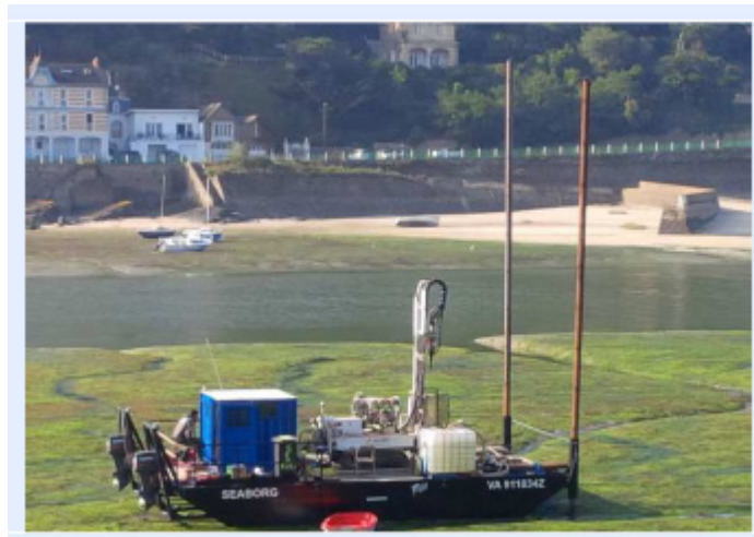
Exemple de ponton flottant
