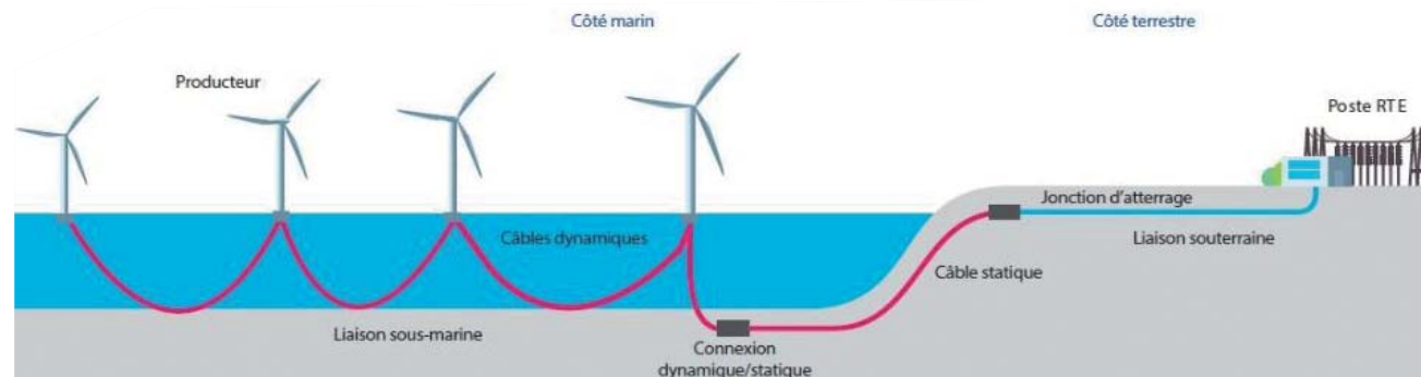
Principe de raccordement entre le projet pilote et le réseau de transport d'électricité
